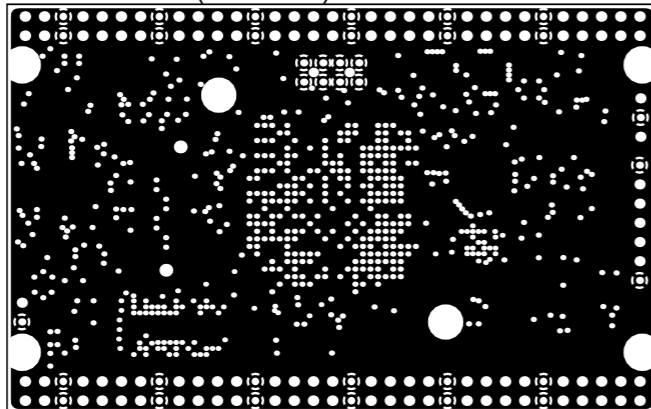
InternalPlane1 (Scale 1:1)
