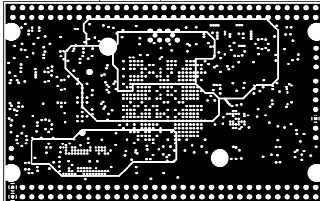
InternalPlane3 (Scale 1:1)
