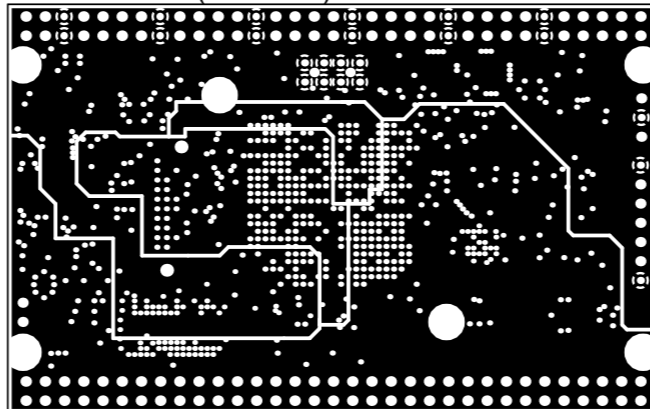
InternalPlane4 (Scale 1:1)
