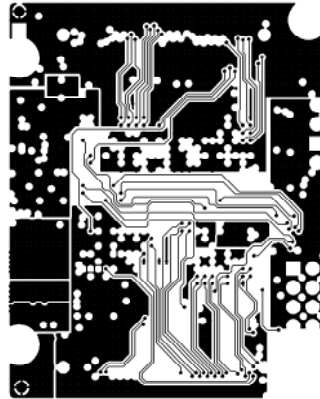
MID LAYER1
