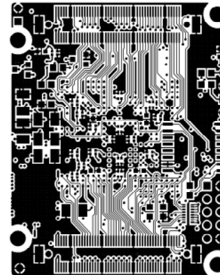
BOTTOM LAYER
