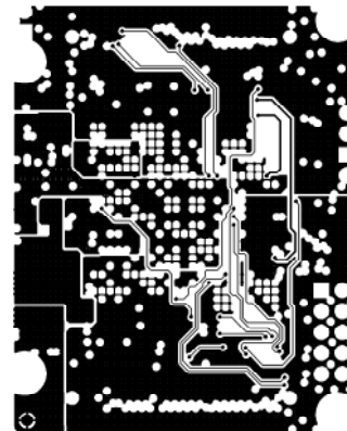
MID LAYER2
