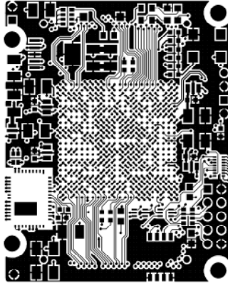
TOP LAYER
