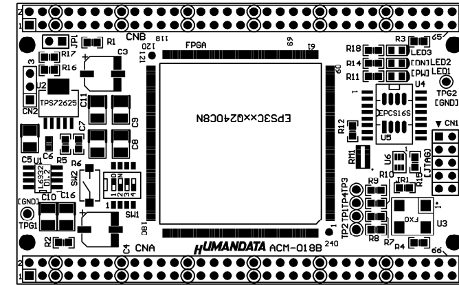
部品面
