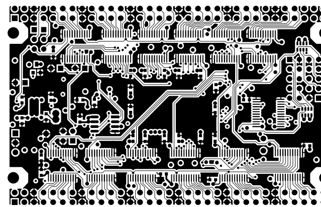
BOTTOM LAYER
