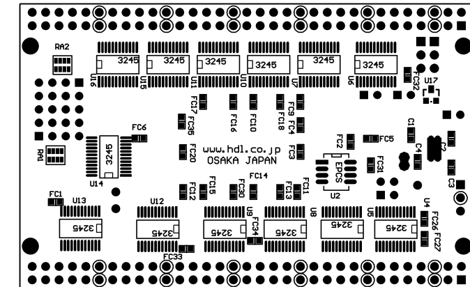
はんだ面
