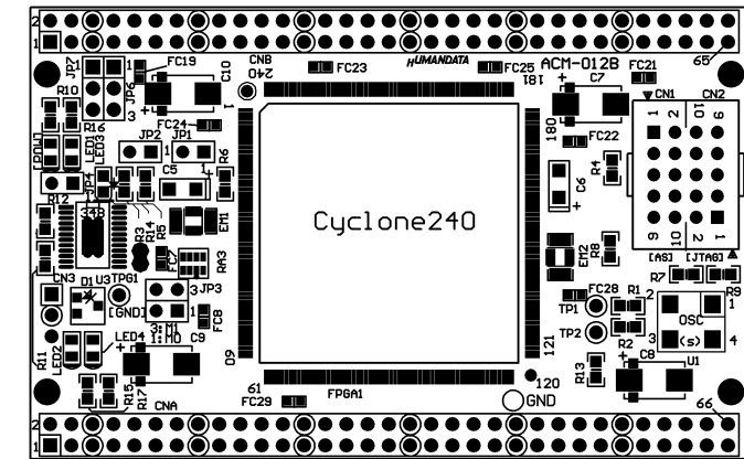
部品面
