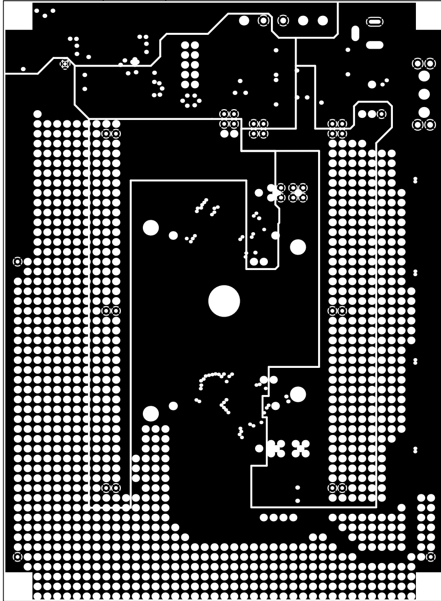
InternalPlane2 (Scale 1:1)
