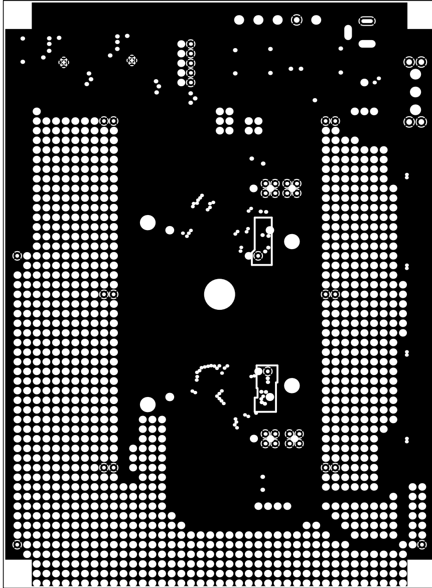
InternalPlane1 (Scale 1:1)
