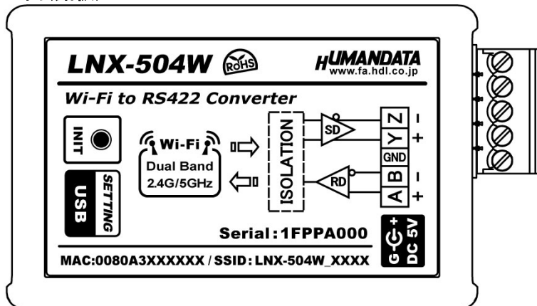
上面(銘板)
