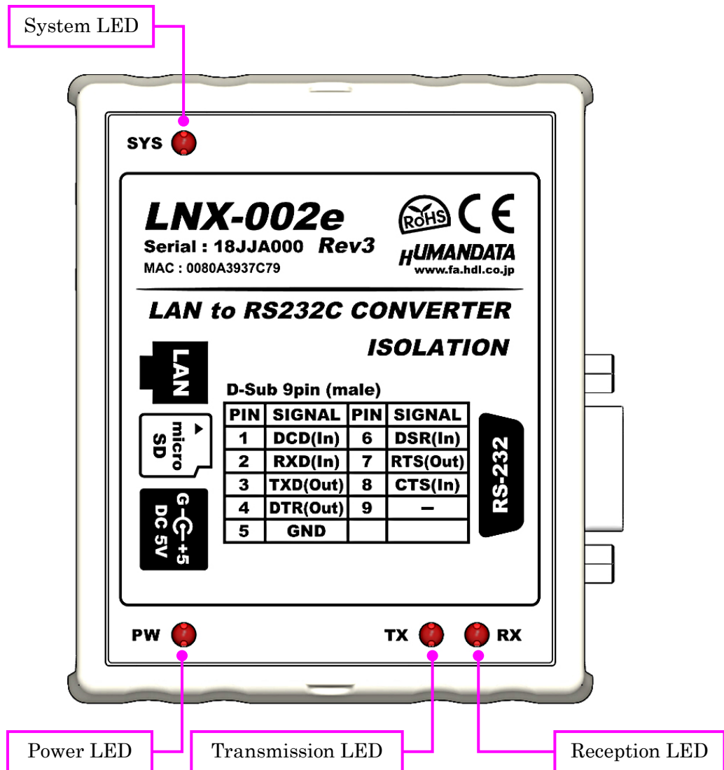
TOP Side
