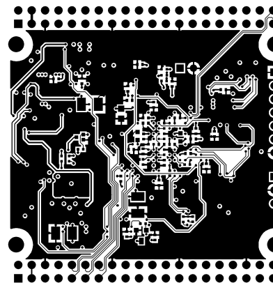
BOTTOM LAYER
