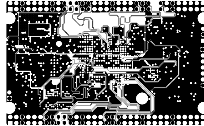
MID LAYER2
