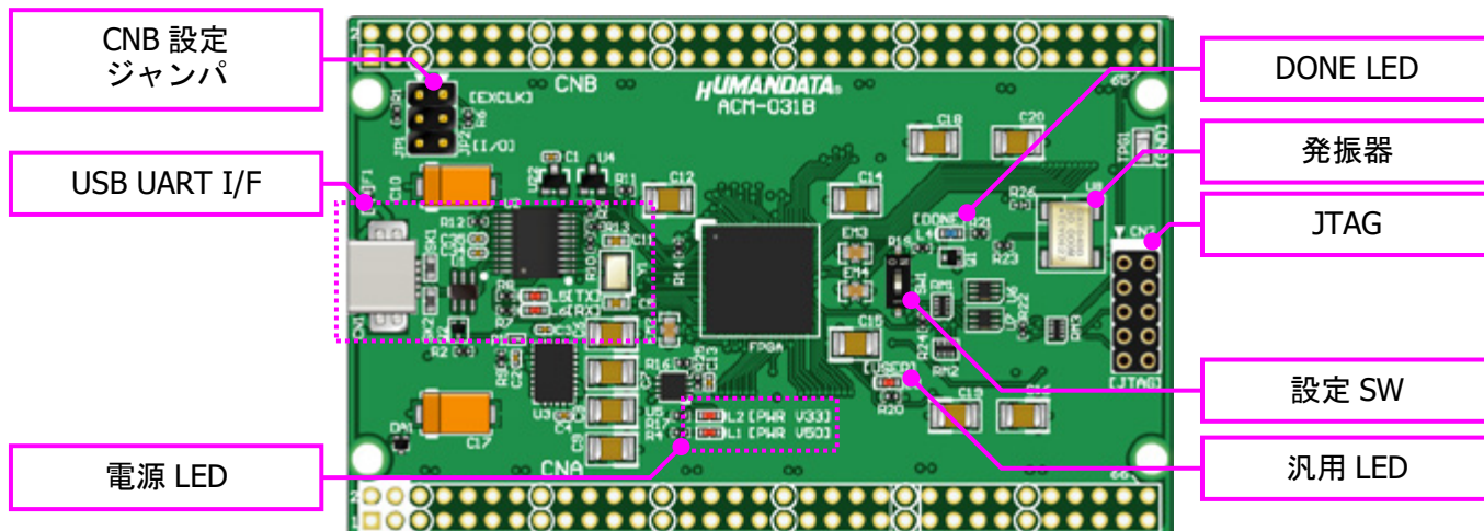
部品面
