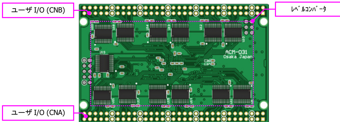
はんだ面
