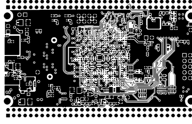
BOTTOM LAYER
